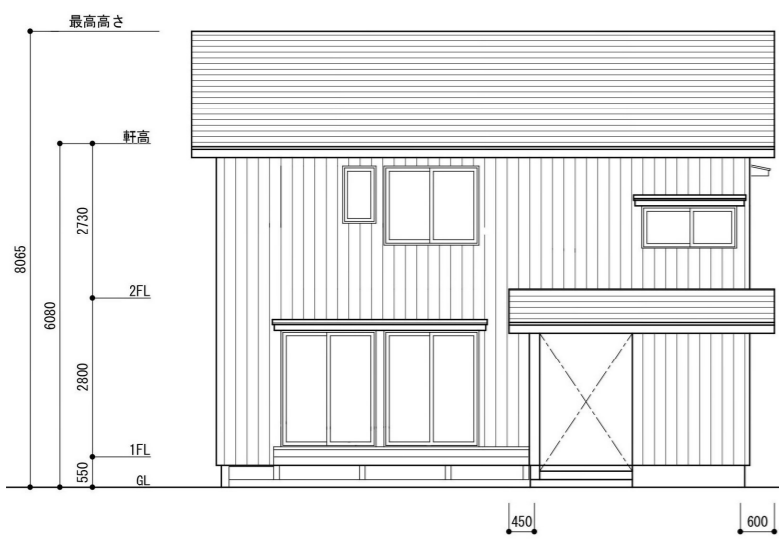
南立面図
