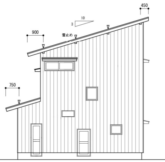
東立面図
