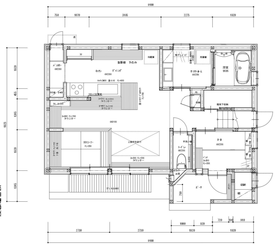
1階平面図
