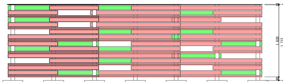
東側立面図 S=1/40
