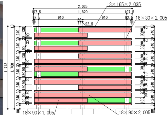
東側①立面図 S=1/40
