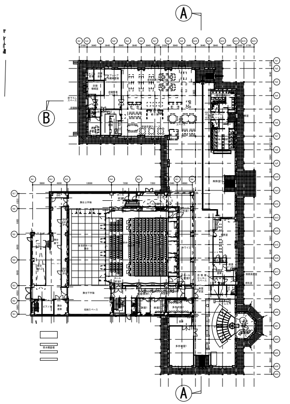
1階平面図 S=1:1000
