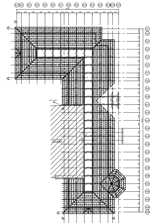
木造棟梁伏図 S=1:1000
