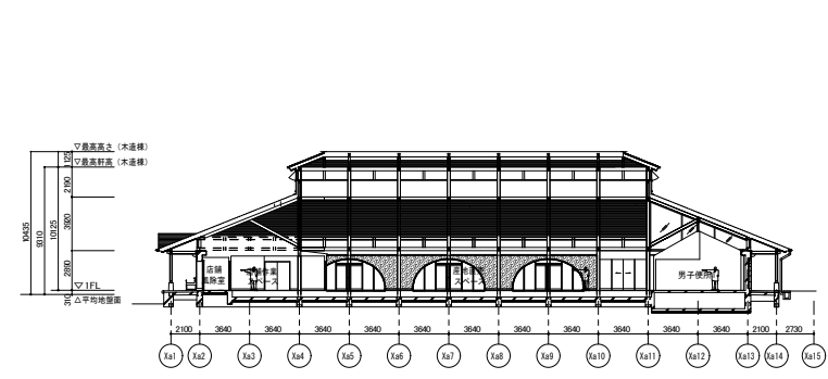
B-B断面詳細図 S=1:600
