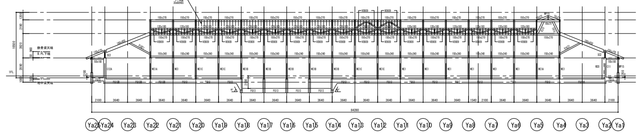
木造棟軸組図 S=1:600
