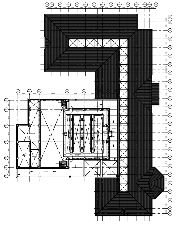
3階平面図 S=1:1000
