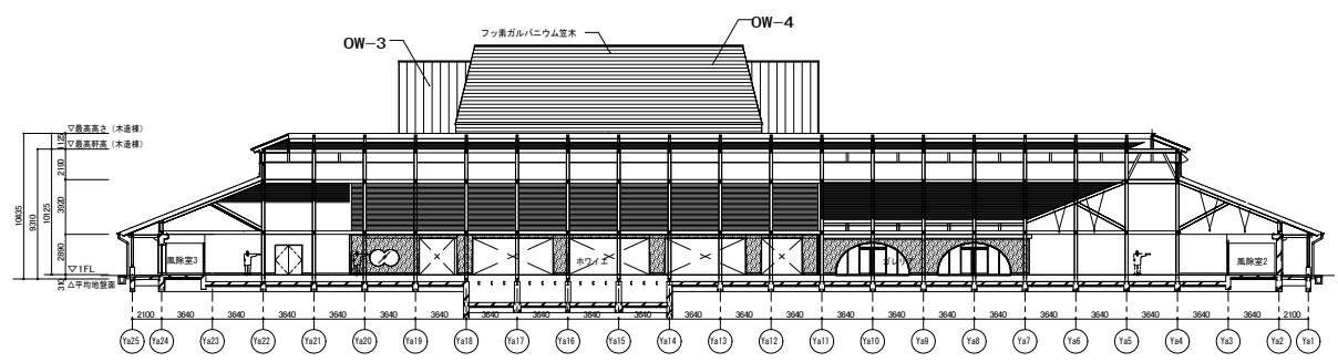
A-A断面詳細図 S=1:600
