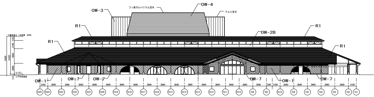
東側立面図 S=1:600
