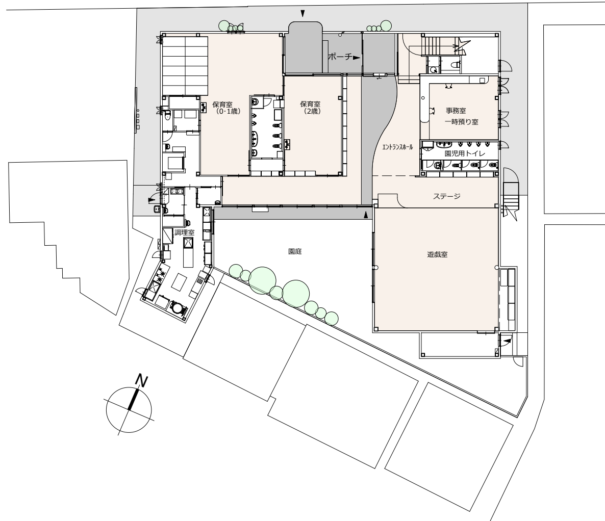
1階平面図 兼 配置図 S=1/300
