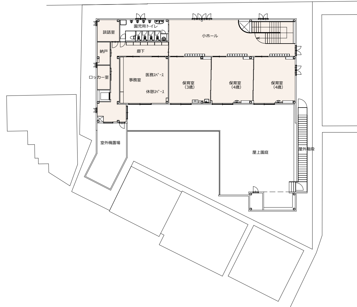
2階平面図 兼 配置図 S=1/300
