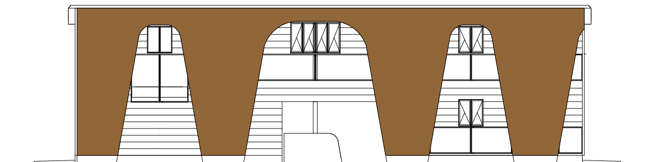
北面 立面図 S=1/200
