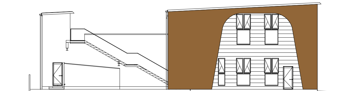
東面 立面図 S=1/200
