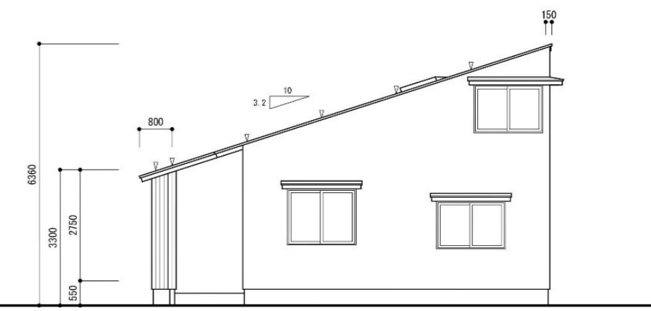
東 立面図
