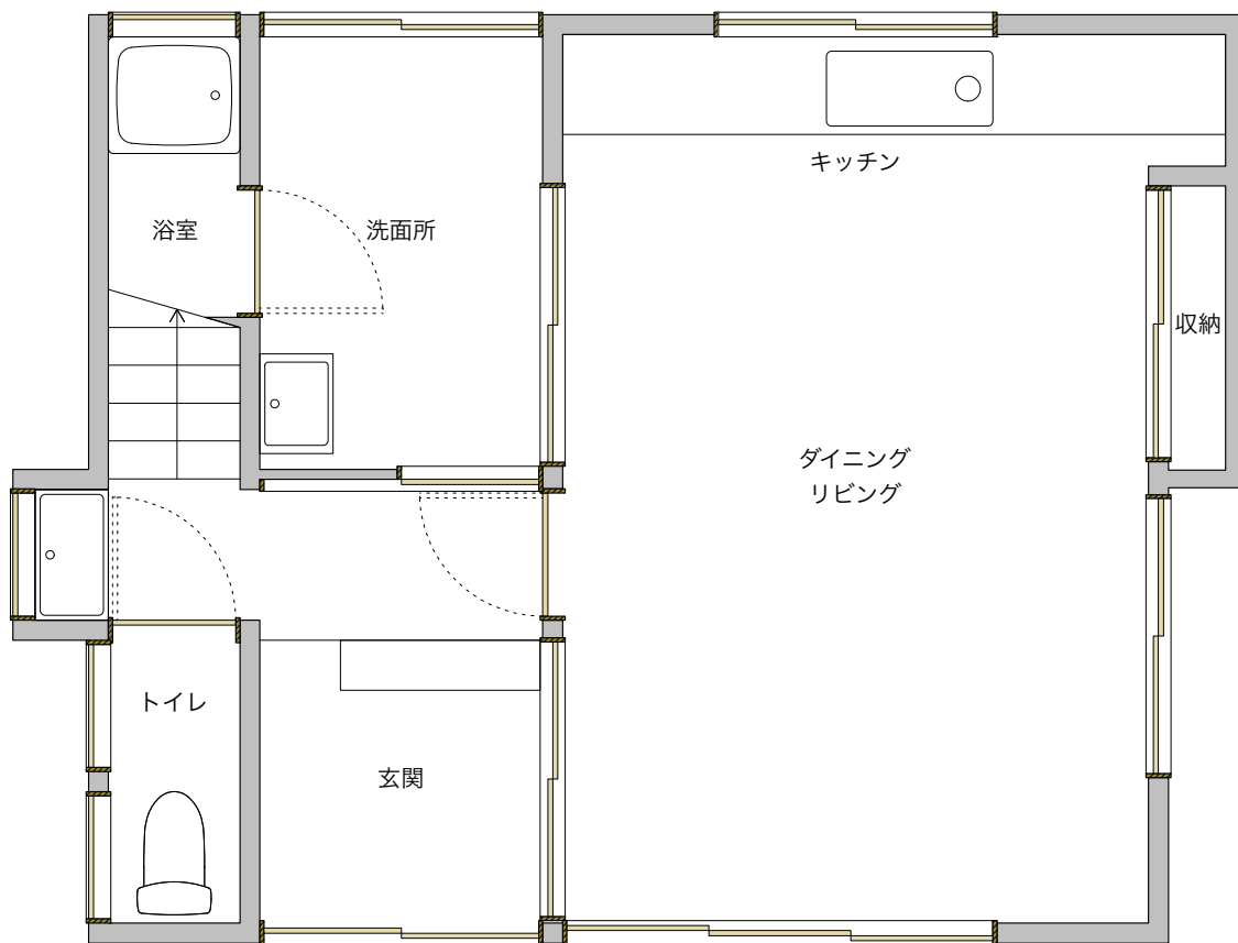
改装後
