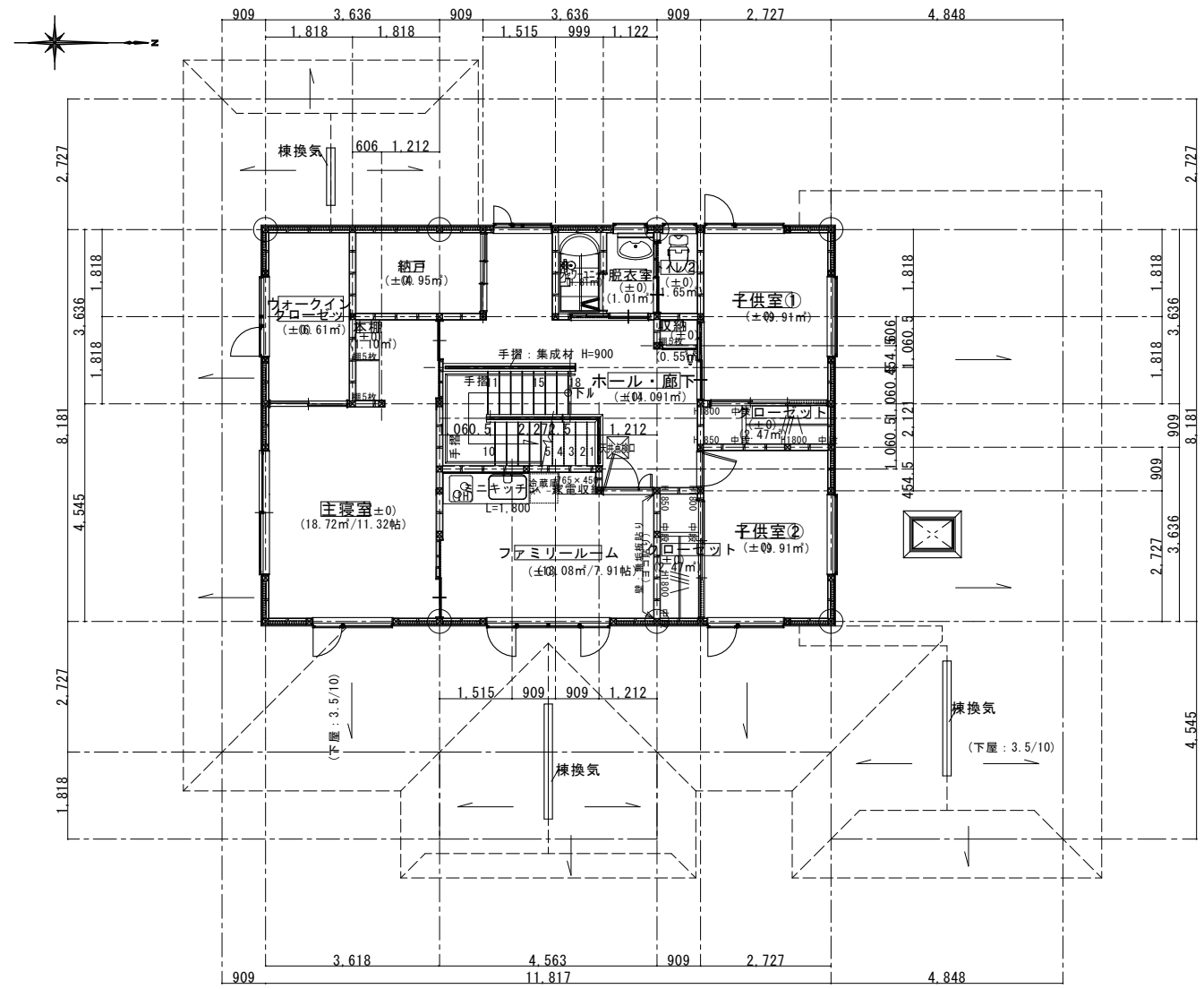
2階平面図
