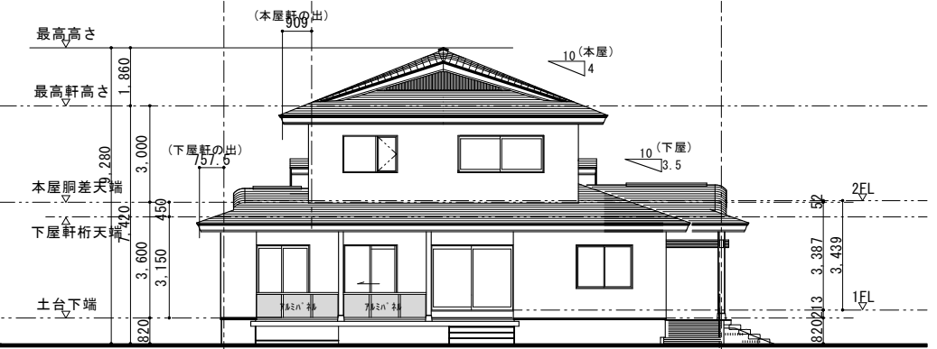
南立面図
