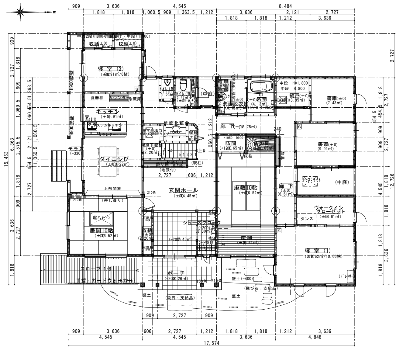
1階平面図
