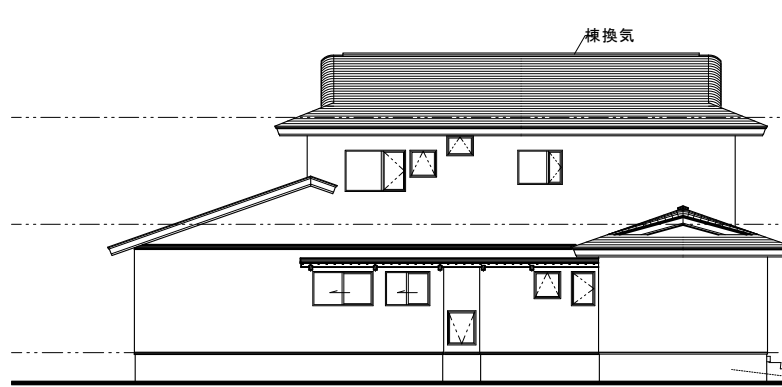
西立面図
