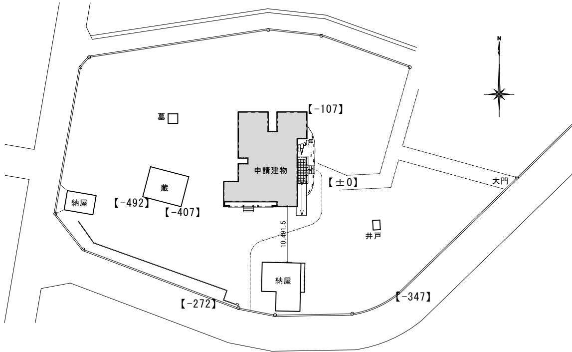
敷地、配置図
