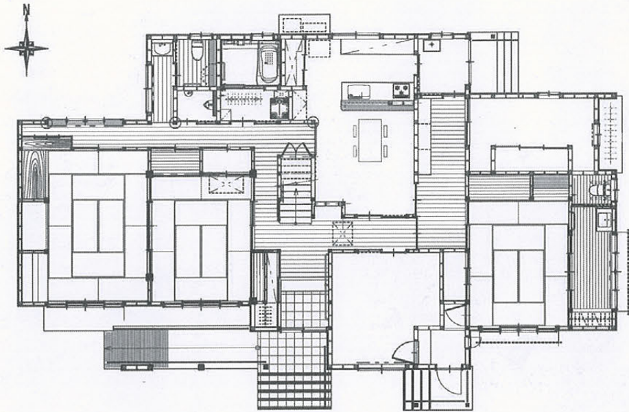
1階平面図
