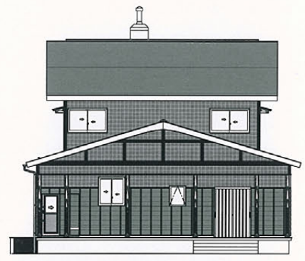
東側立面図
