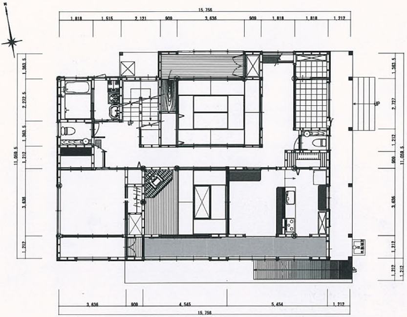
1 階平面図
