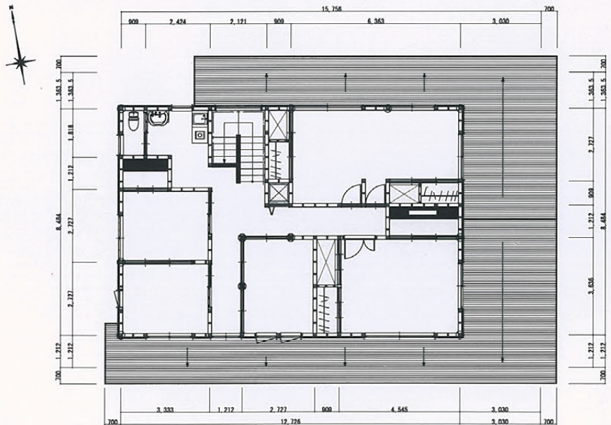
1 階平面図
