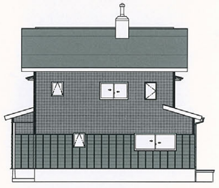
西側立面図
