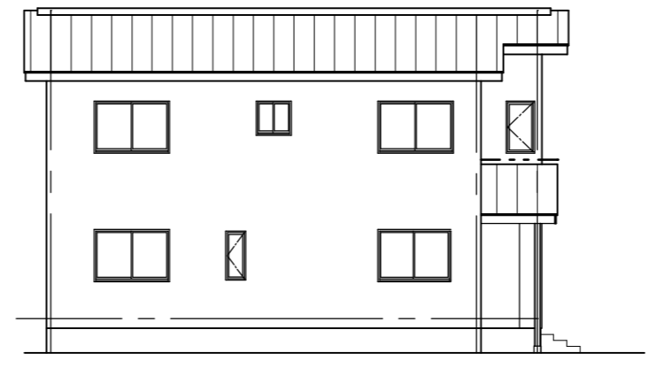
南側立面図 S=1/150
