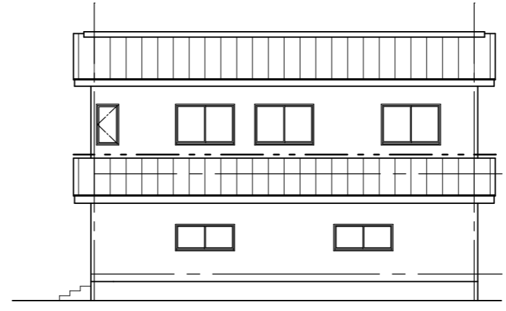
北側立面図 S=1/150
