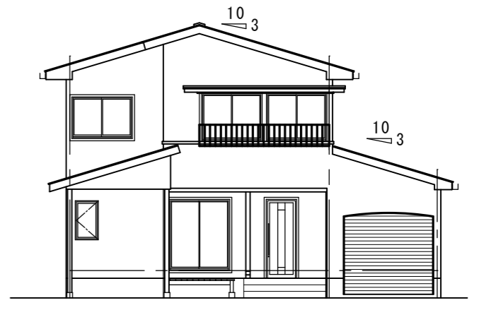
東側立面図 S=1/150
