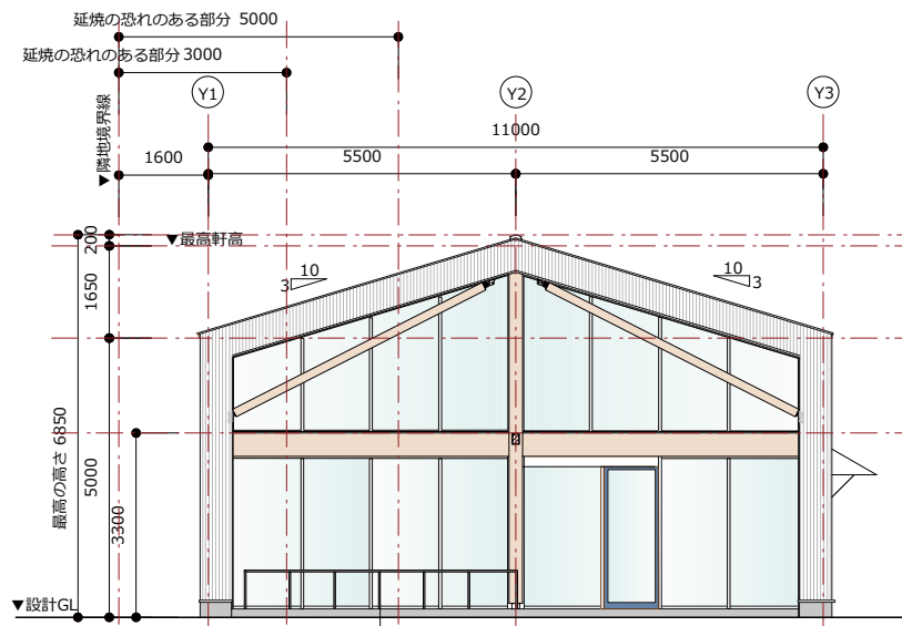
南立面図
