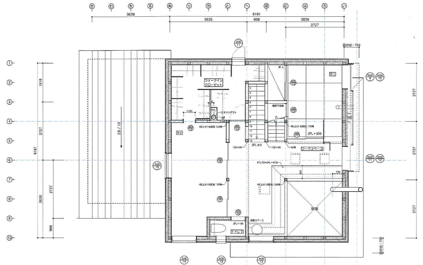
平面詳細図-1階
