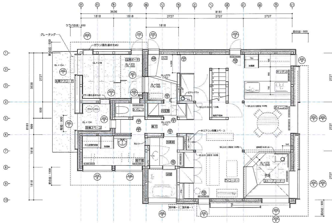
平面詳細図-1階
