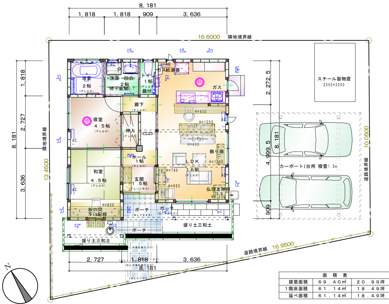
平面詳細図 1階
