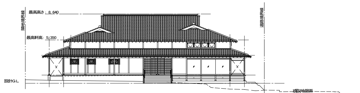
立面図 S=1:200
