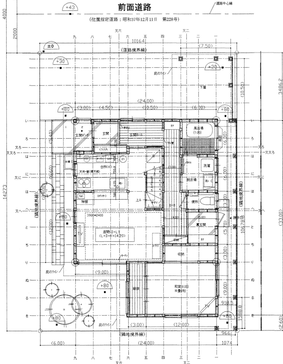
1階平面図
