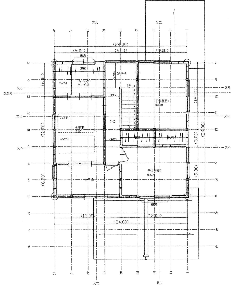
2階平面図
