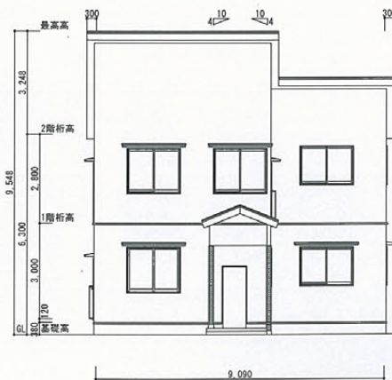
南立面図 S-1/150
