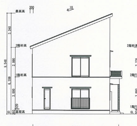
西立面図 S-1/150
