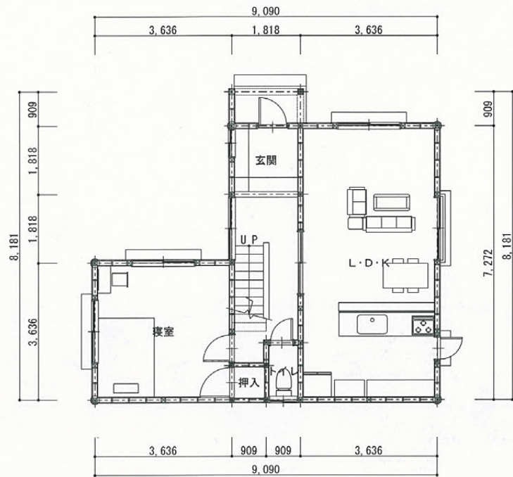
1階平面図 S-1/100
