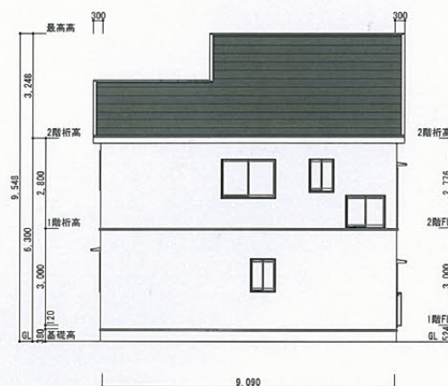
北立面図 S-1/150
