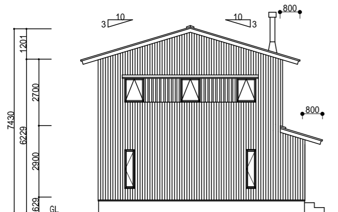
西側 立面図 S = 1/150
