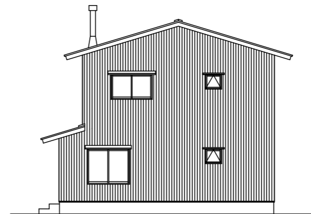
東側 立面図 S = 1/150
