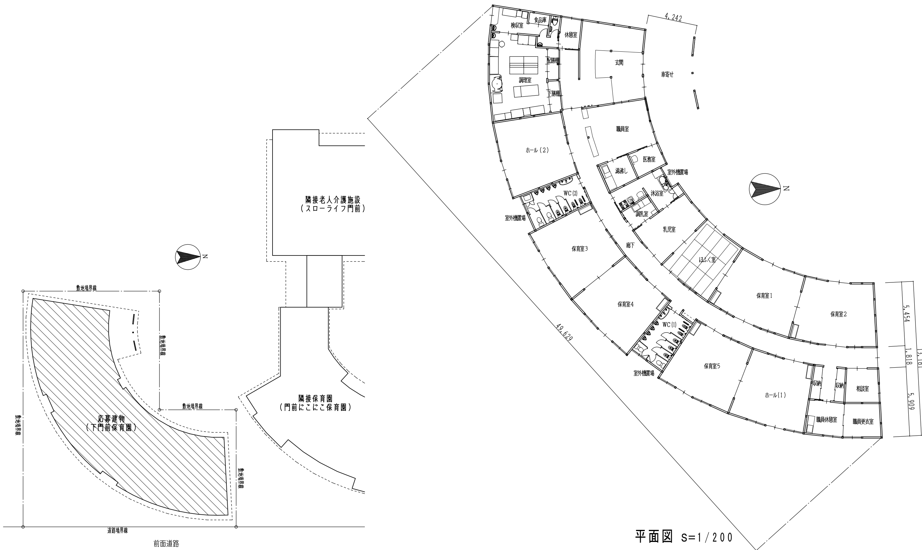
配置図 s=1/400
